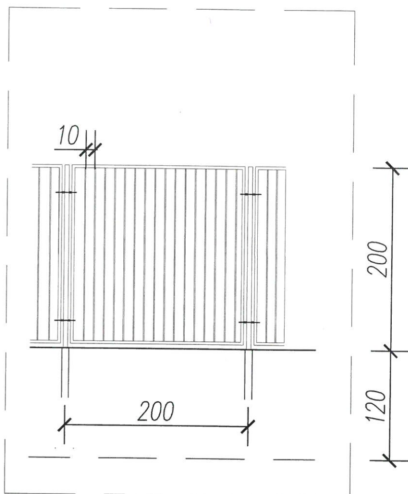
SCHEMAT PRZĘŚŁA
